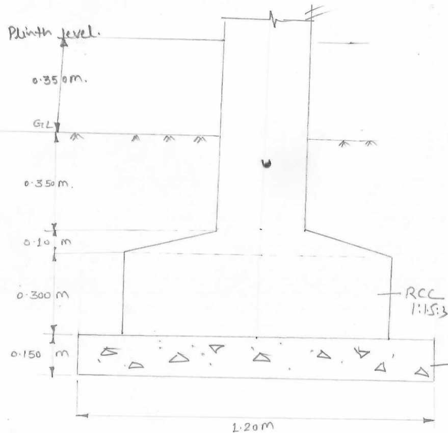
ELEVATION
